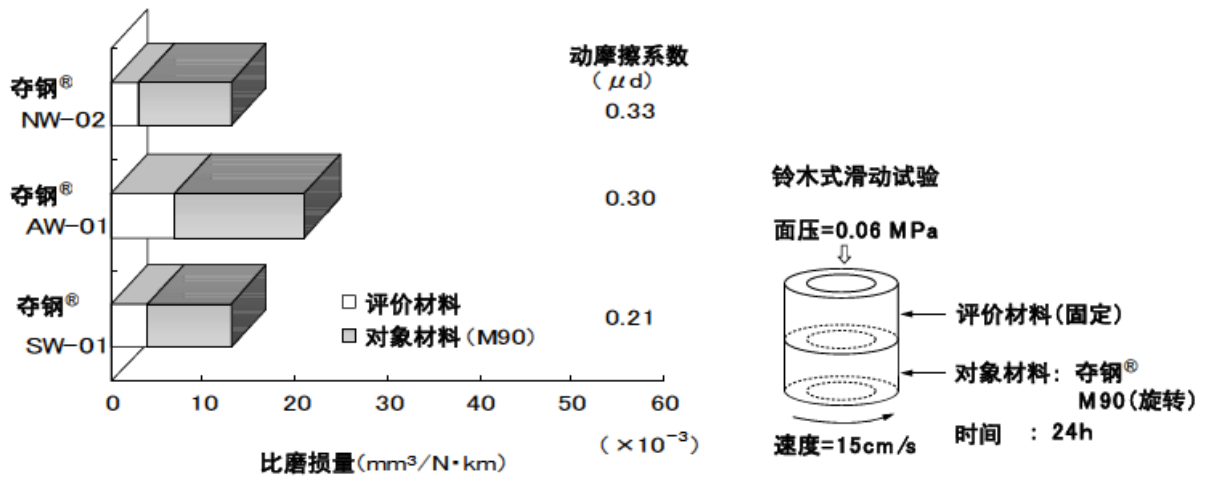
图 1-4 中负荷 低温 (-10℃) 下的摩擦磨损特性（铃木式滑动）
