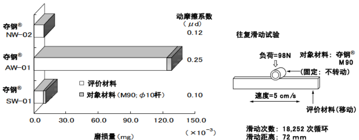
图 1-5 高负荷 摩擦磨损特性（往复滑动）
